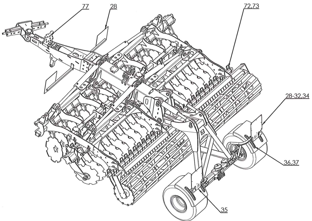
Ciężka brona ścierniskowa U-671 Standard wersja składana hydraulicznie półzawieszana Heavy stubble harrow U 671 Standard hydraulically folded trailed version
