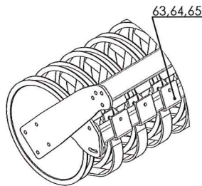
Wał U-ring Ø540 U-ring roller Ø540
