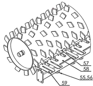
Wał Packer Ø460/550 Packer roller Ø460/550
