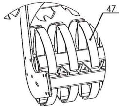
Wał sprężynowy Ø550/470 Spring roller Ø550/470
